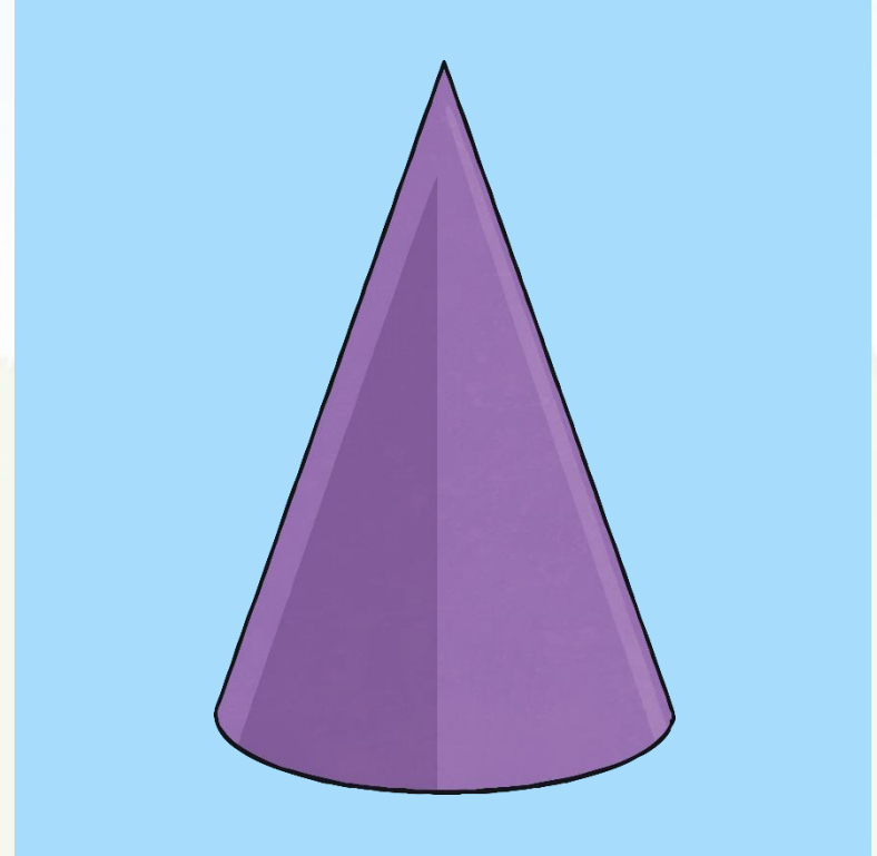
Cone
