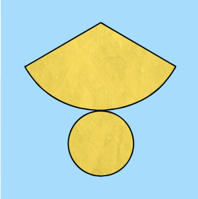
Cone
